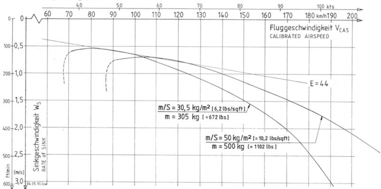
ASW 24 Flugleistungspolaren
